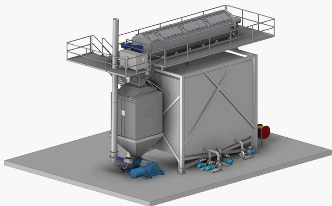
Sistema de pesagem e drenagem de peixes – simples
